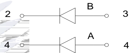
Fig.1-4 Polarity 极性
