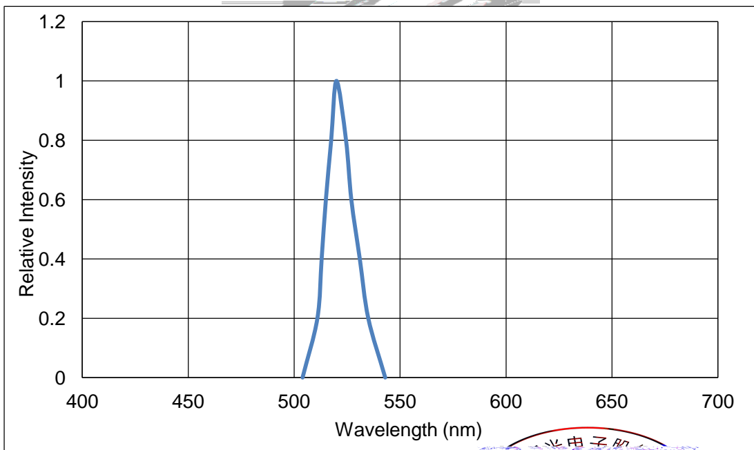
Fig 1-11 Relative Intensity Vs Wavelength (Ta=25°C) 相对光谱与波长关系曲线
