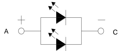
Fig.1-4 Polarity 极性
