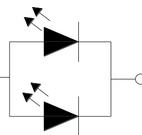
Fig.1-4 Polarity 极性
